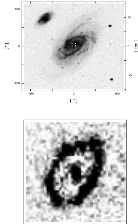
Fig. 1. Arriba: Imagen (DSS) de la galaxia Seyfert NGC 1241 y su compañera NGC 1242. Abajo: Emisión \text{Pa}\alpha en los dos kpc ( 7.8'' ) centrales de NGC 1241, el continuo de la banda H fue sustraído. Nótese la barra nuclear y la estructura de brazos "leading" en emisión.
